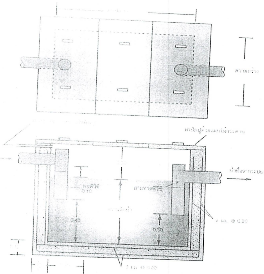
ขนาดมาตรฐานบ่อดักไขมันแบบสร้างในที่
