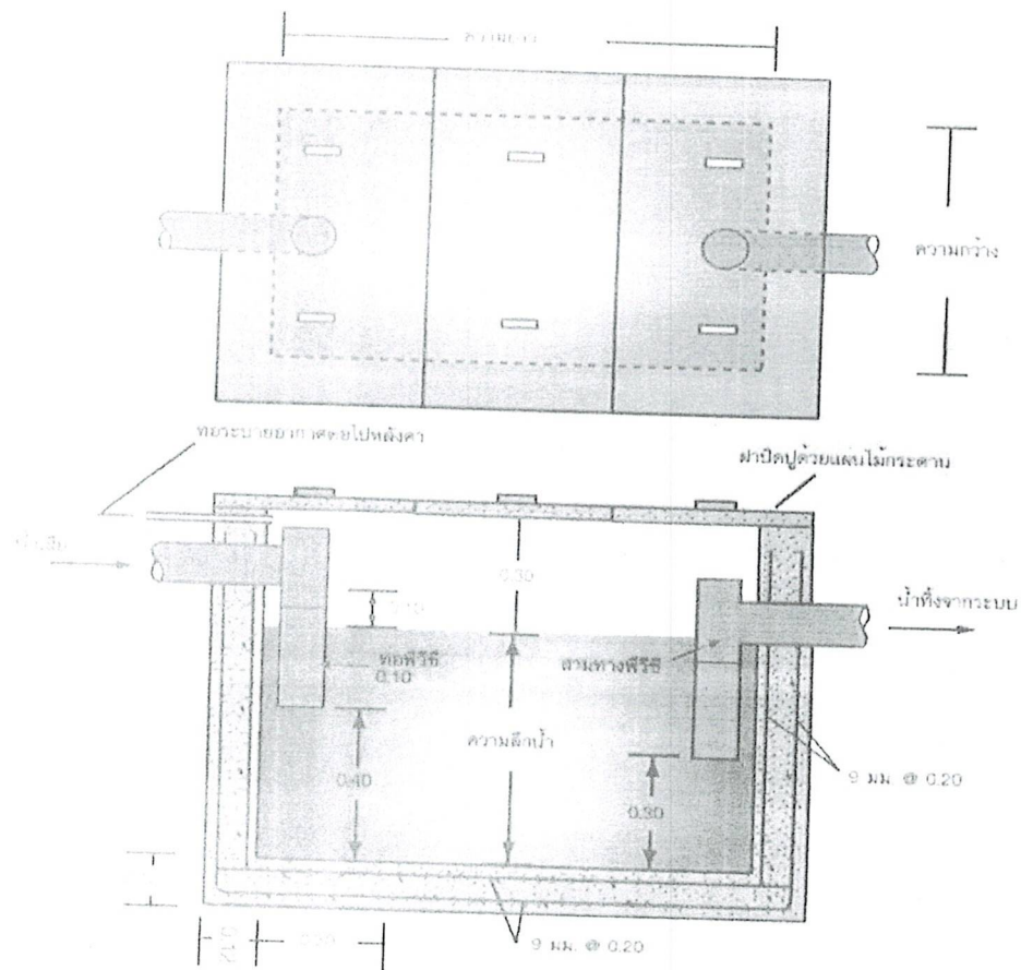
ขนาดมาตรฐานบ่อตกไขมันแบบสร้างในที่
